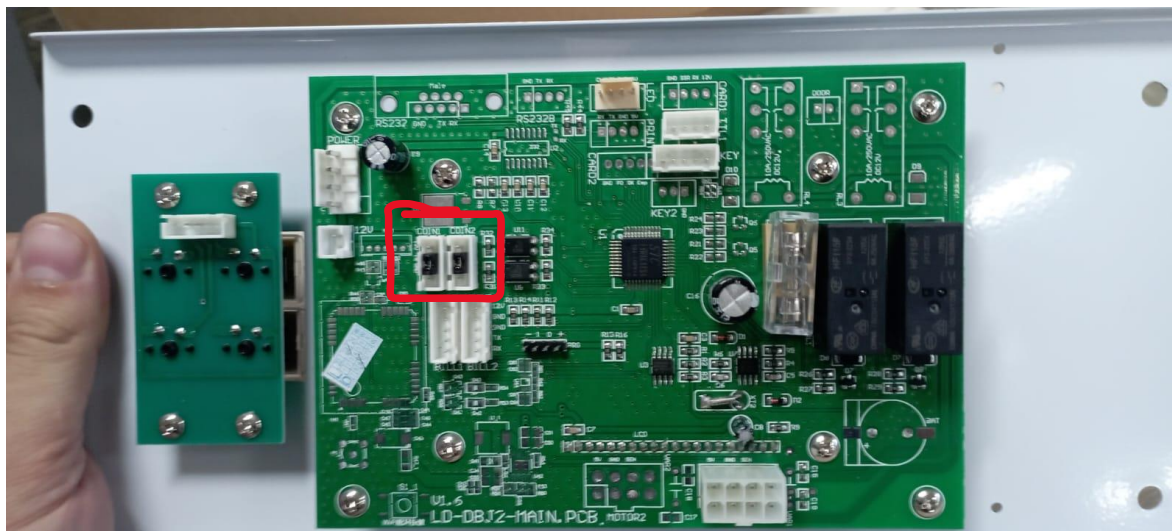
Figura 19 – Placa de controle da máquina trocadora de fichas
